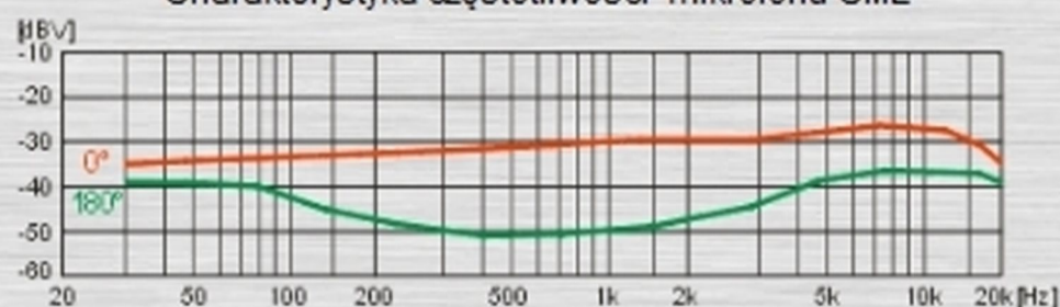
Charakterystyka częstotliwości mikrofonu CML
