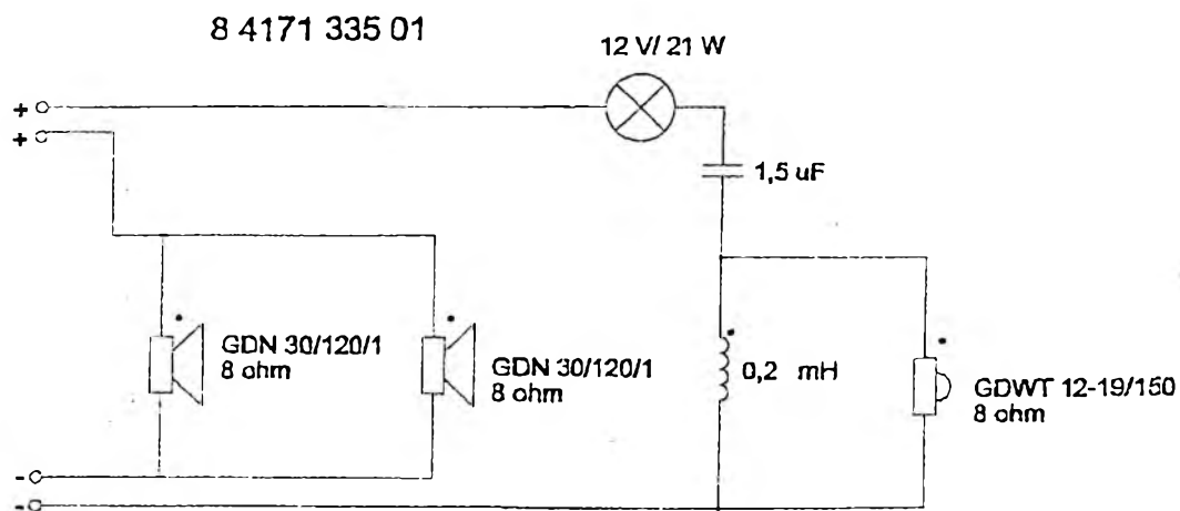
SCHEMAT ZWROTNICY ELEKTRYCZNEJ
