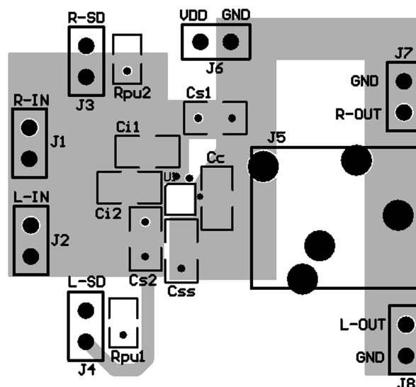
Bottom Layer
