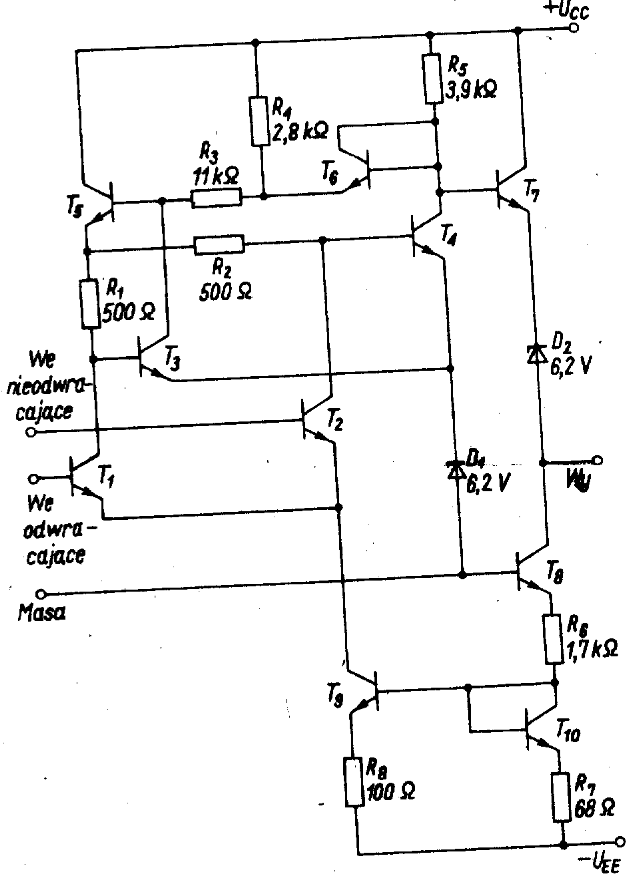
Schemat elektryczny komparatora \mu A 710
