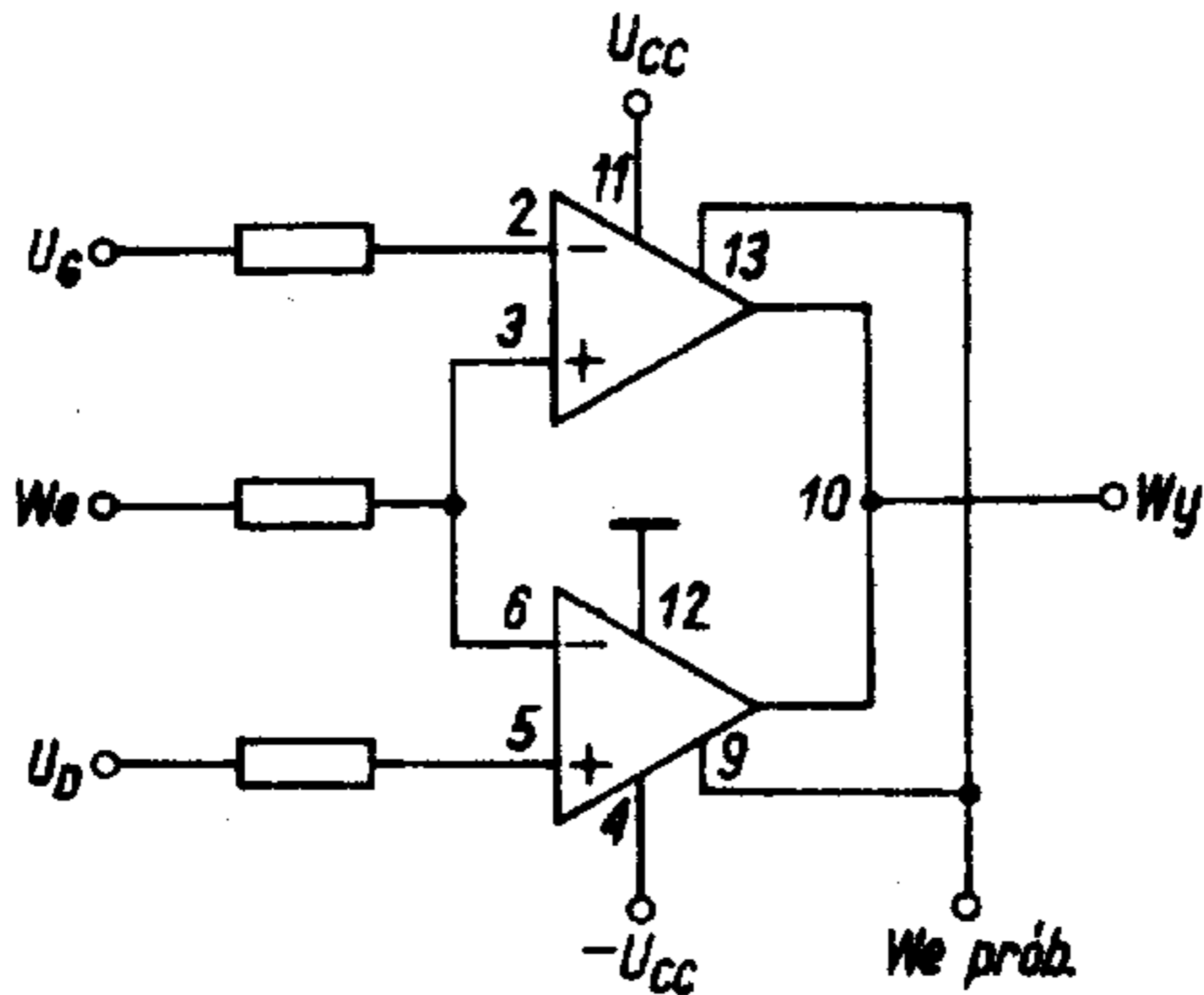
●5.13B● Schemat funkcjonalny podwójnego komparatora \mu A 711
