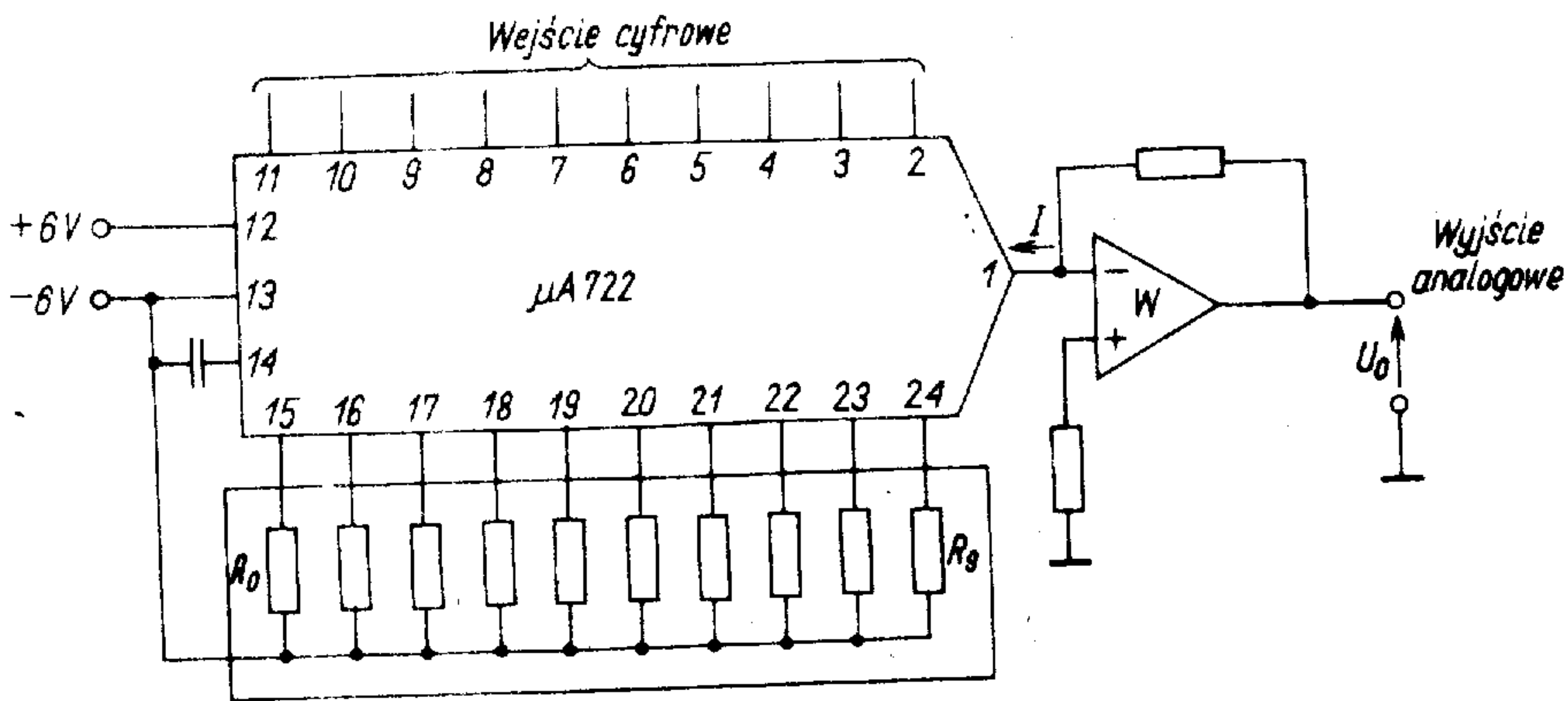
● 5.19D ● Schemat przetwornika c/a zbudowanego z zastosowaniem układu \mu A 722
