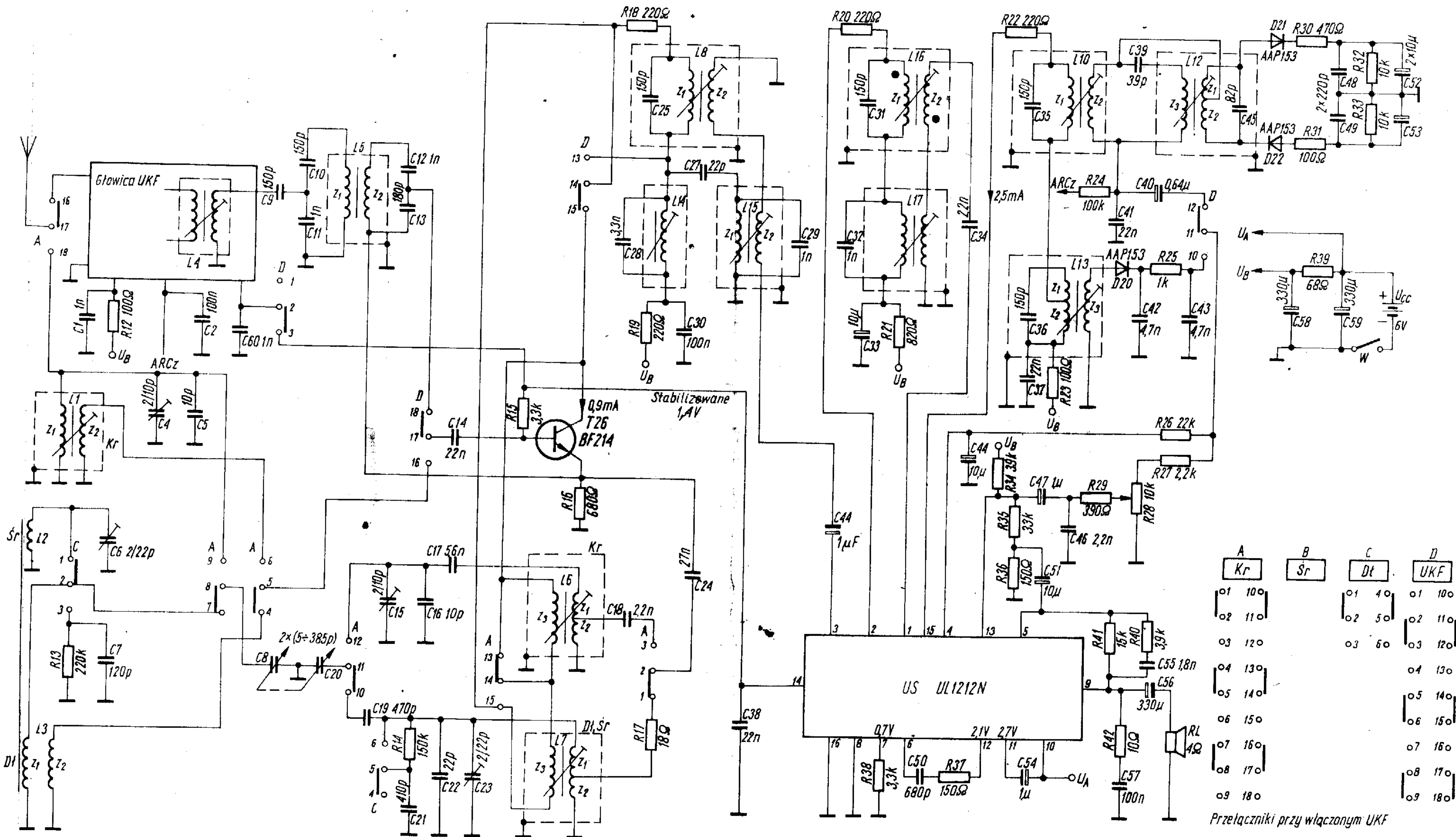
Rys. 2. Schemat odbiornika radiowego z układem UL1212N
