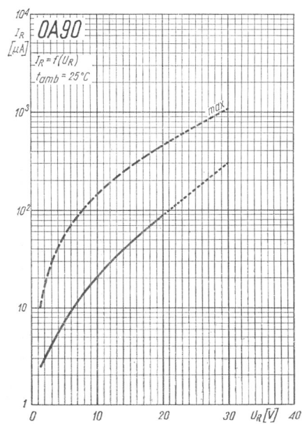
Rys. 2-161. Charakterystyki prądu wstecznego diody
