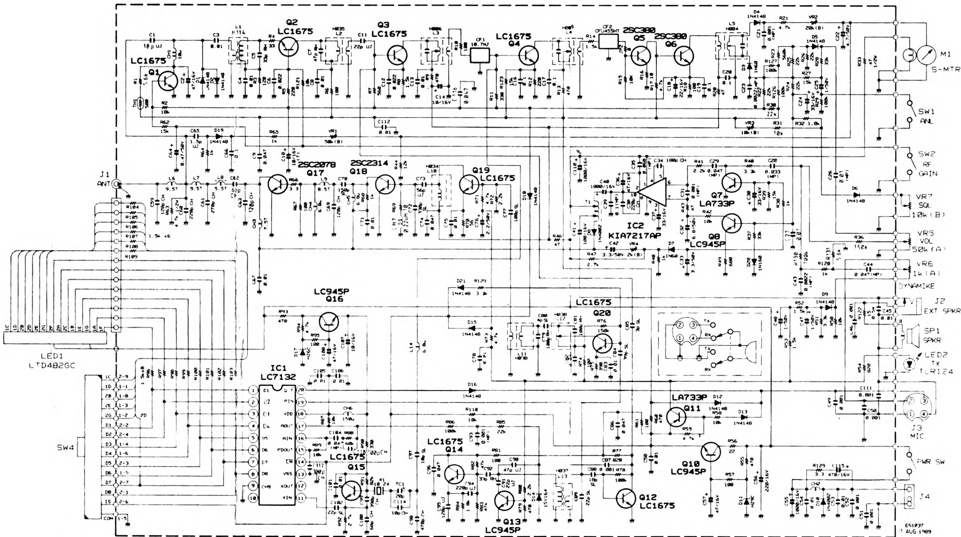
Schemat ideowy radiotelefonu Cobra 21 LTD Classic
