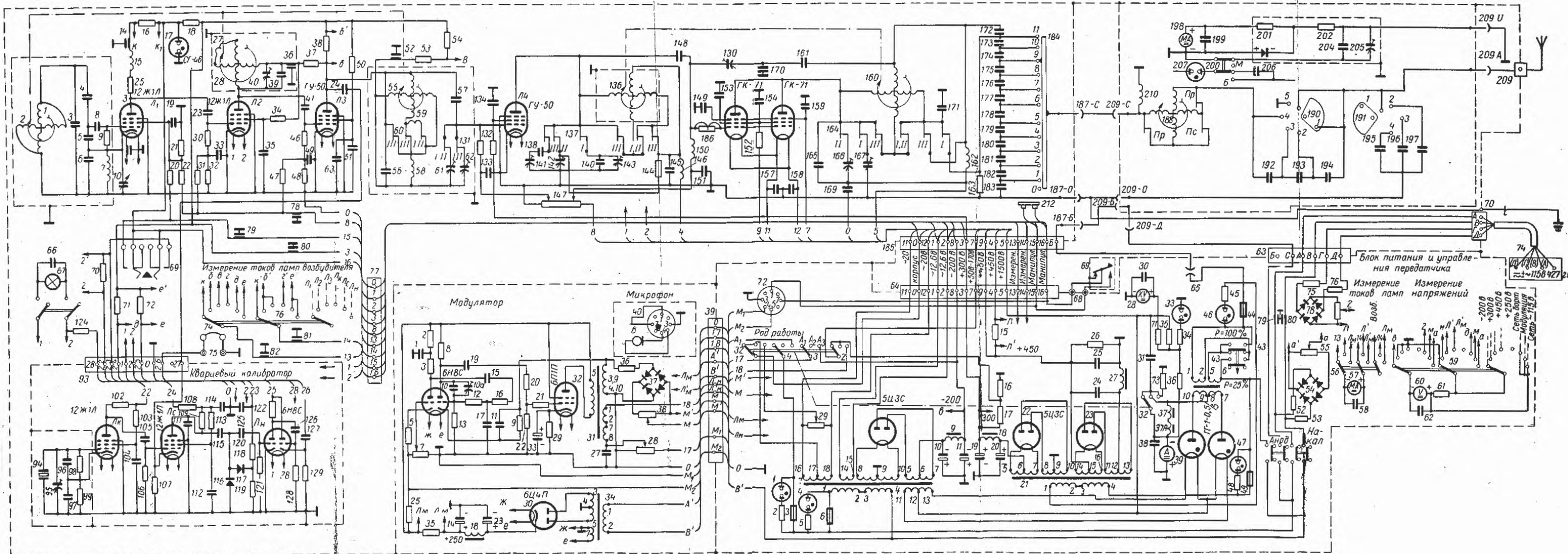
Принципиальная схема передатчика "Блесна КВМ"
