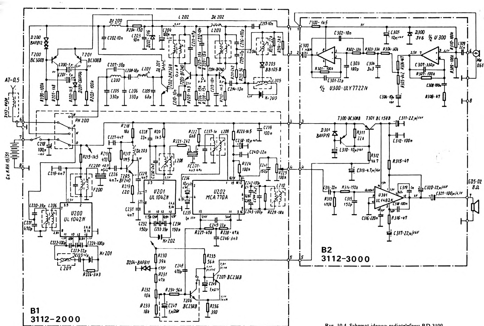
Rys. 10.4. Schemat ideowy radiotelefonu RD 3109
