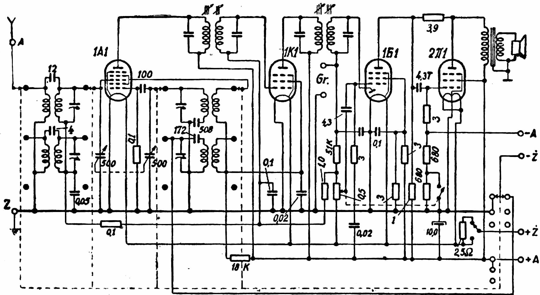
Schemat odbiornika radzieckiego Tajin B-2
