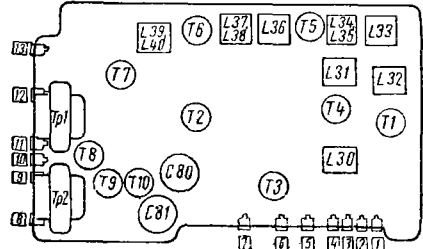
Расположение элементов на печатной плате
