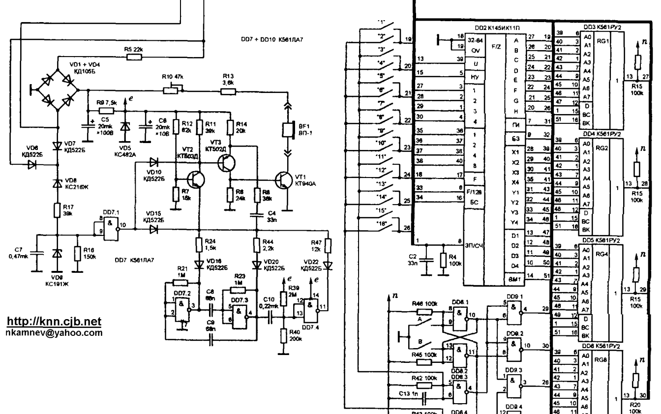
Телефонный аппарат VEF TA-32
